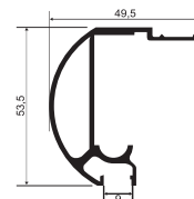
1021/B - Trilho Superior para box
