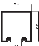
1030P - Trilho Stanley (pesado)
