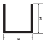
1018 - Perfil lateral 16x16mm para 10mm
