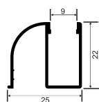
1016/C - Trilho inferior para box
