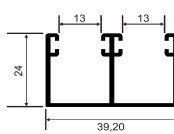
1034D/R - Trilho inferior duplo p/ 8mm
