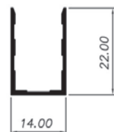
1019B - Perfil lateral para 10mm
