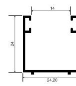
1034/S - Trilho inferior simples 10mm
