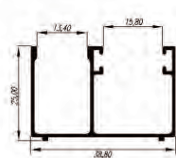
1034 - Trilho inferior para 10mm
