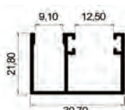
1034R - Trilho inferior para 8mm
