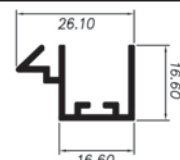
1018T - Perfil lateral c/ engate para 1570
